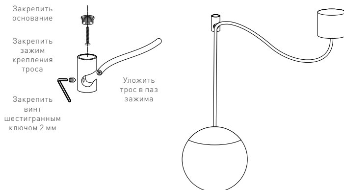
Рис. 1. Установка подвеса
