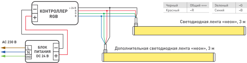
Схема 2. Подключение нескольких светодиодных лент «неон» с одной стороны. Арт. 047041
