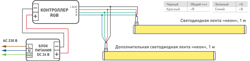
Схема 1. Подключение нескольких светодиодных лент «неон» с одной стороны. Арт. 047199
