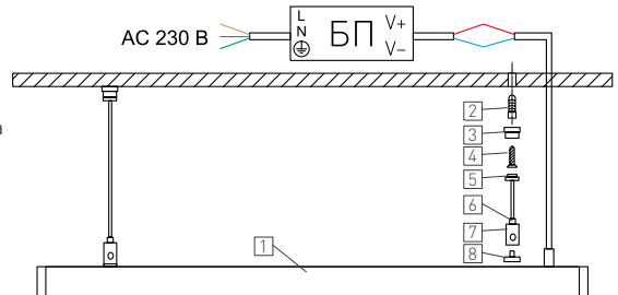
Рис. 2. Монтаж светильника
