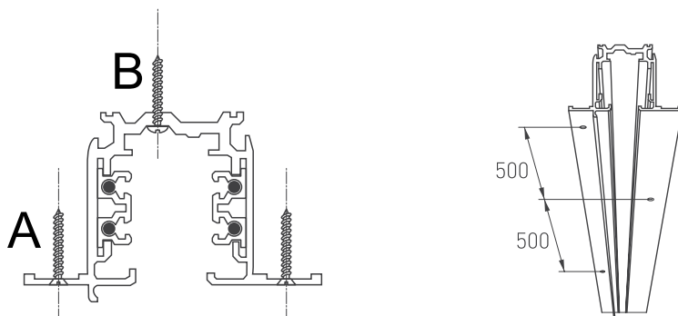
Рис. 2. Установка шинопровода в нишу
