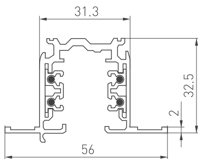
Рис. 1. Чертеж встраиваемого шинопровода
