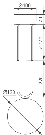
Рис. 1. Чертеж и габаритные размеры
