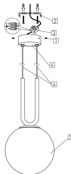
Рис. 2. Установка и подключение светильника
