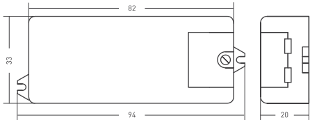
Рисунок 1. Размеры блока управления.
