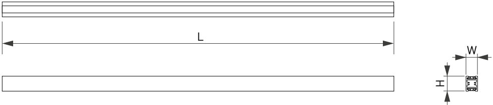
Рис. 1. Чертеж и габаритные размеры прямого шинопровода
