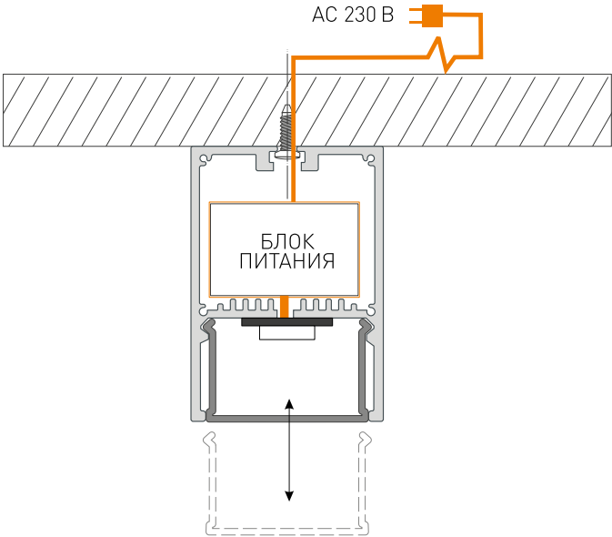
Рис. 1. Установка и подключение светильника
