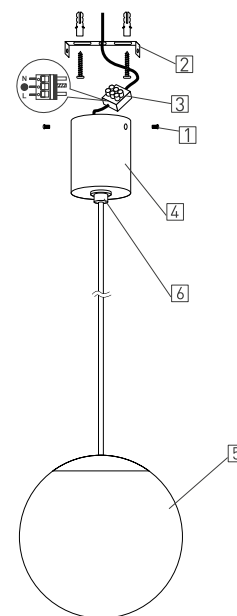
Рис. 2. Установка и подключение светильника
