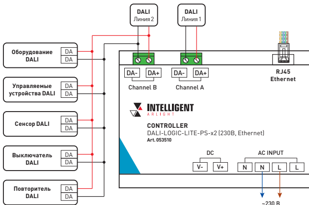
Рис. 1. Подключение контроллера
