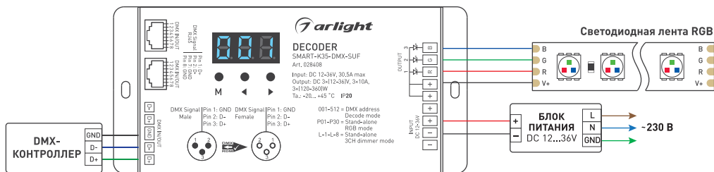
Рисунок 1. Подключение декодера SMART-K35-DMX-SUF
