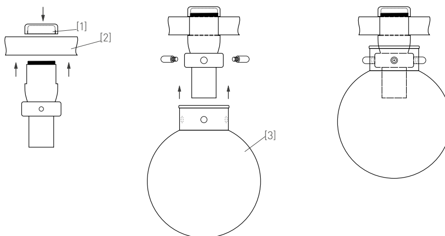
Рис. 2. Установка светильника
