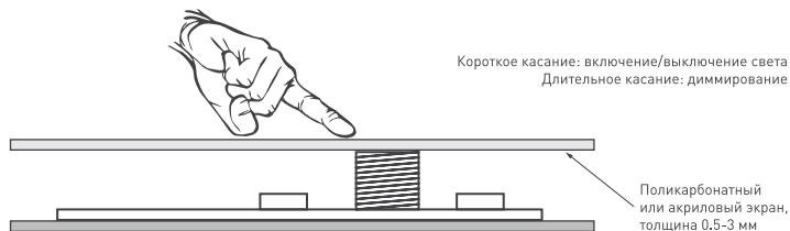
Рисунок 2. Схема установки диммера.
