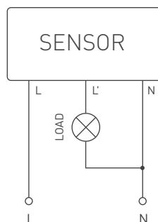
Рис. 3. Схема подключения
