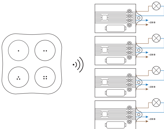
Рисунок 1. Пример управления диммерами панелью TUYA-228-4-RF-WH-SUF
