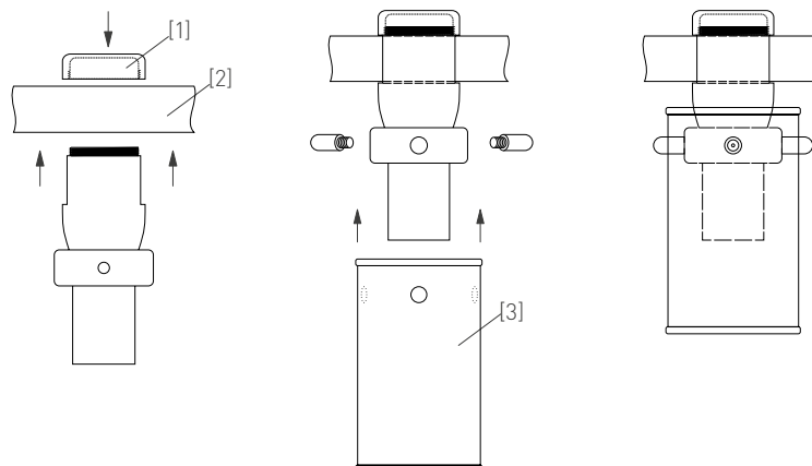
Рис. 2. Установка светильника
