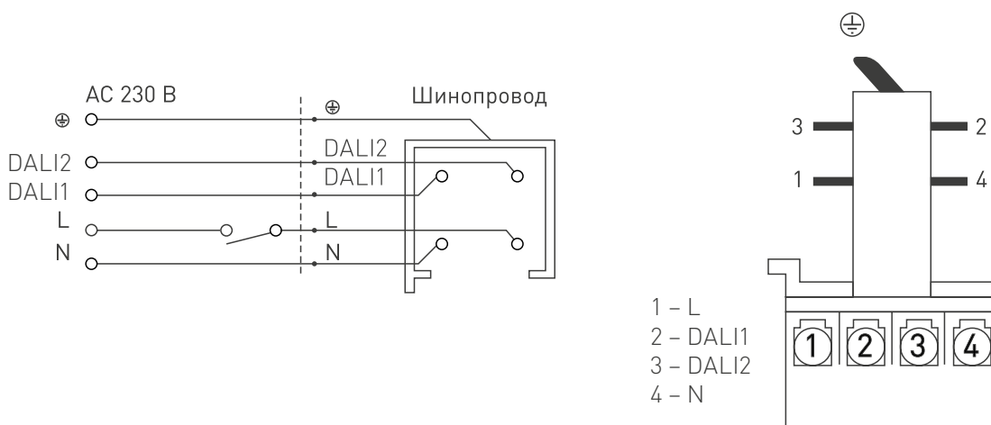
Рис. 2. Схема подключения
