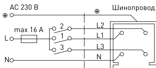
а) 1 фаза, 3 нагрузки, AC 230 В, 16 А, 3.7 кВА
