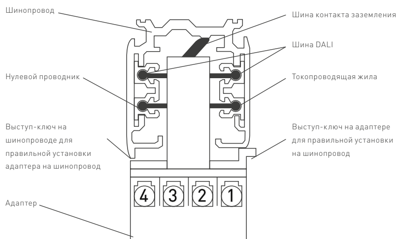
Рисунок 1. Подключение адаптера к шинопроводу
