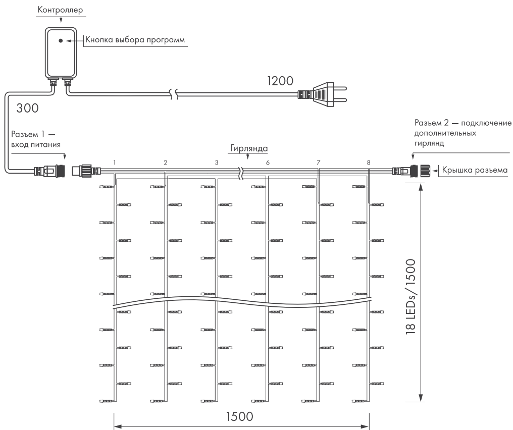
Рисунок 1. Схемы подключения
